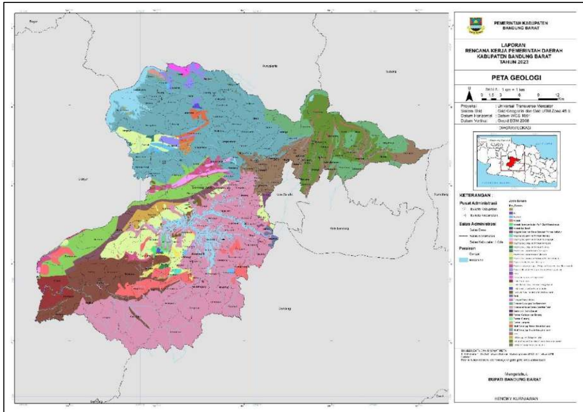
Gambar 2.4 Peta Geologi Kabupaten Bandung Barat
